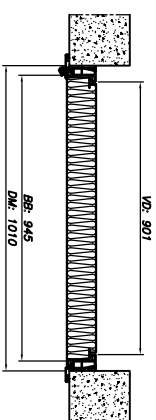
Montage op Beton
