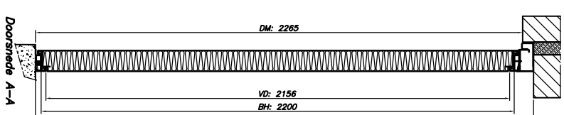
Montage Achter de slag
