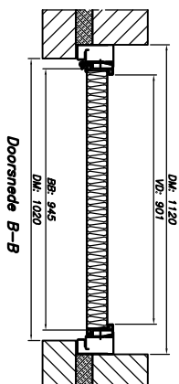
Montage achter de slag
