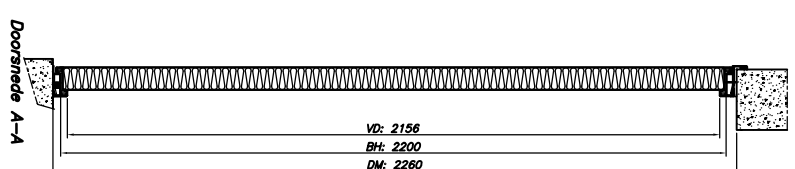
Montage op Beton
