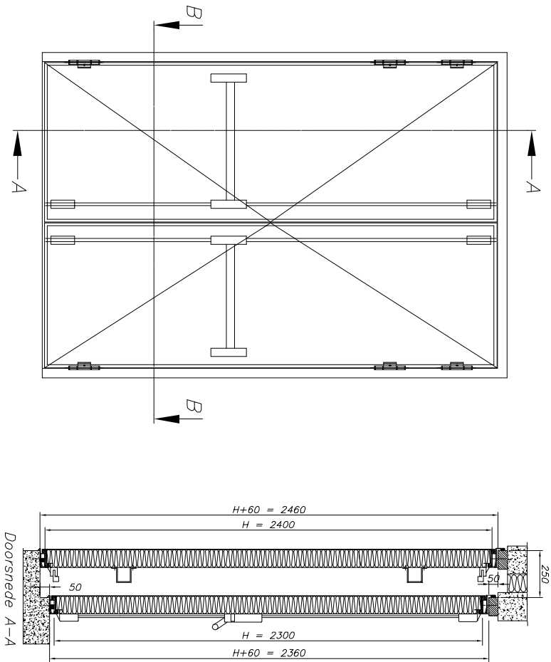
Type: MD56L – Tandemconstructie dubbele deur
