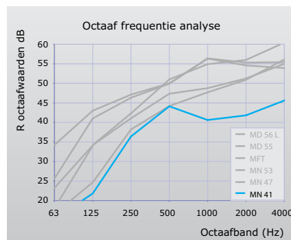
Geluidsisolatiewaarden
